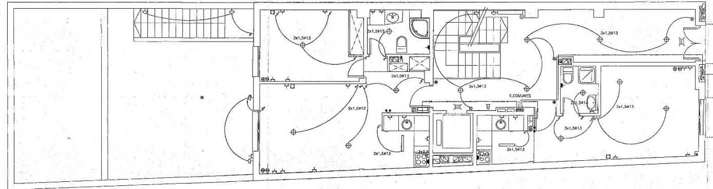
PLANTA BAJA
