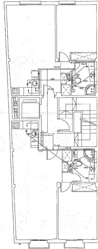
PLANTA SEGUNDA
